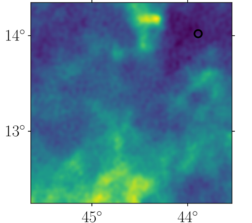
Right ascension
