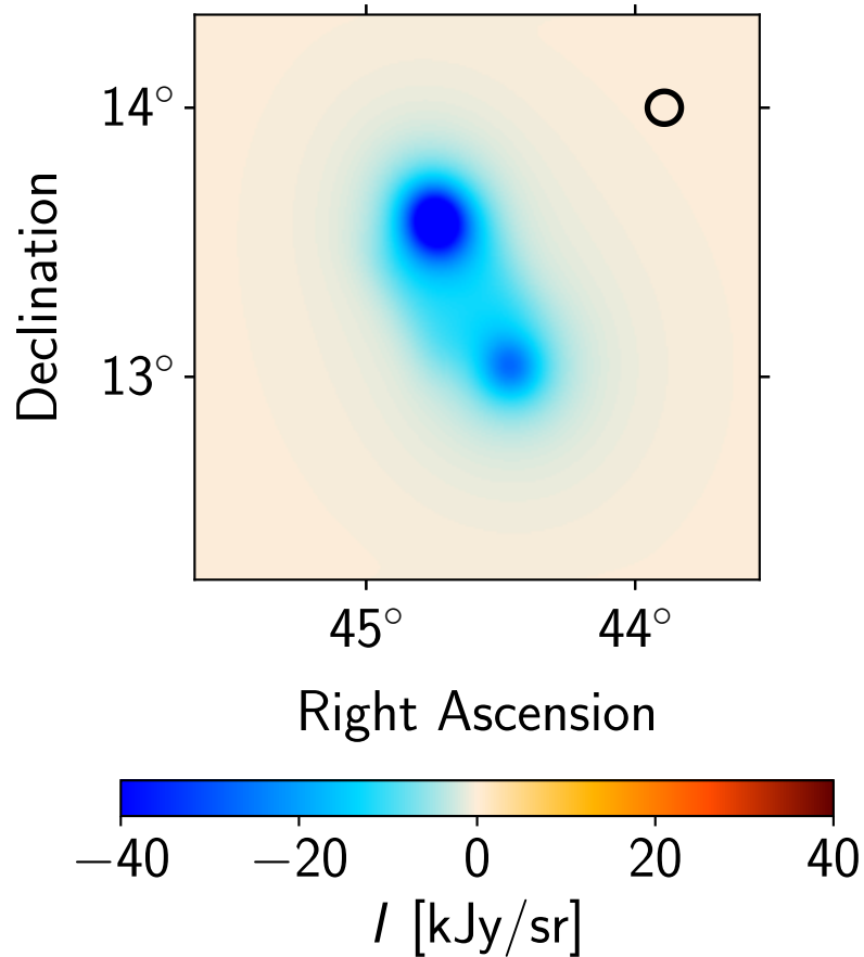
Model: Planck 143 GHz
