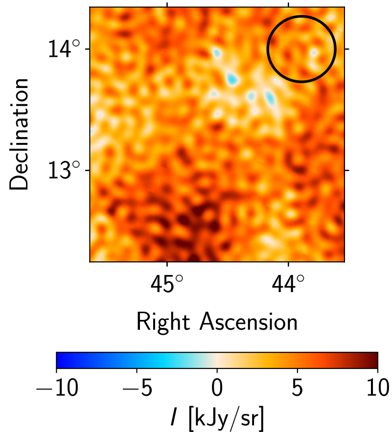
Data: Planck 30 GHz
