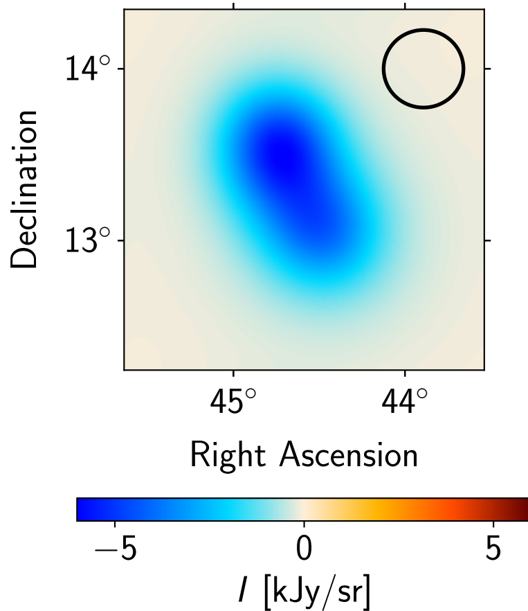
Model: Planck 44 GHz
