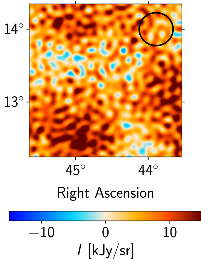
Data: Planck 44 GHz
