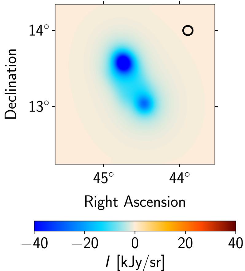
Model: Planck 143 GHz
