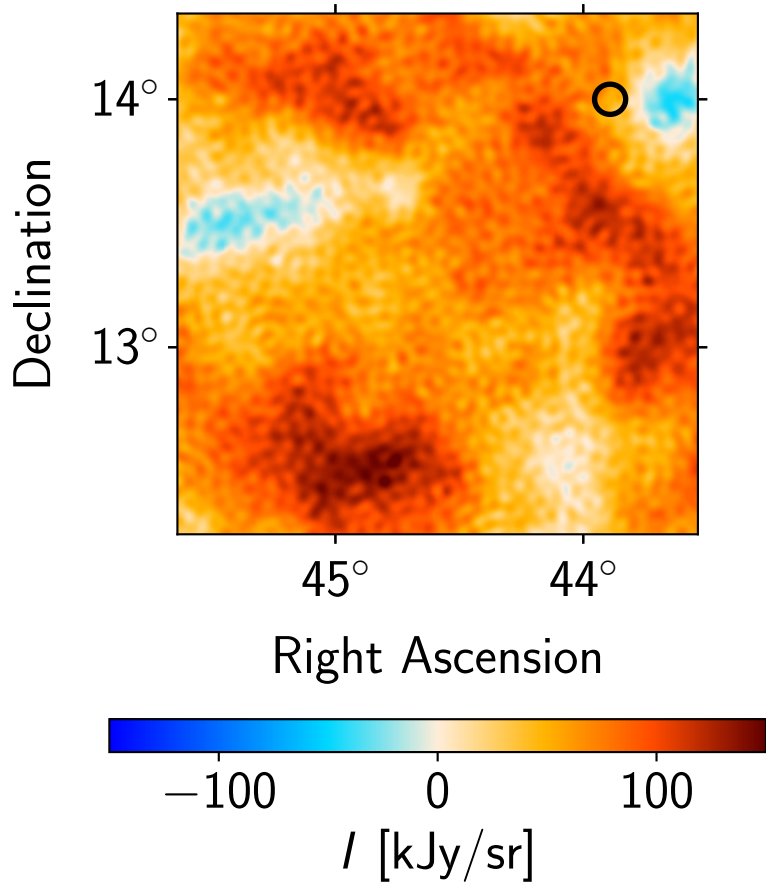
Data: Planck 143 GHz
