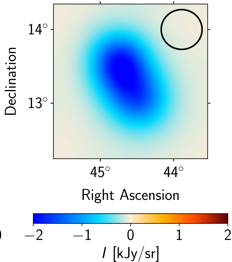
Model: Planck 30 GHz
