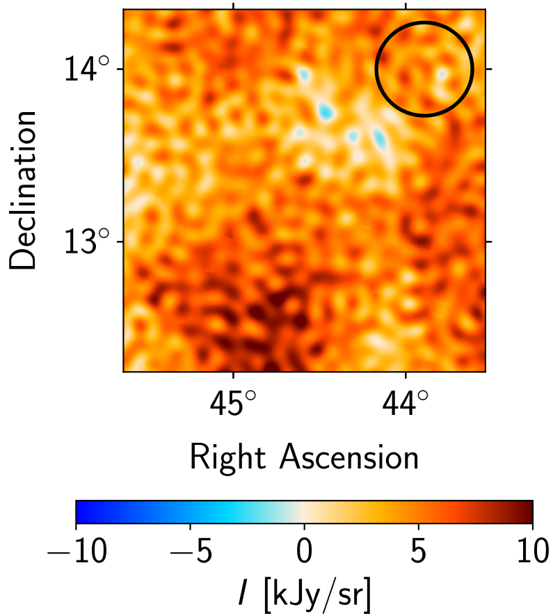
Data: Planck 30 GHz
