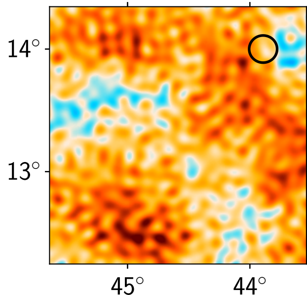
Data: Planck 70 GHz
