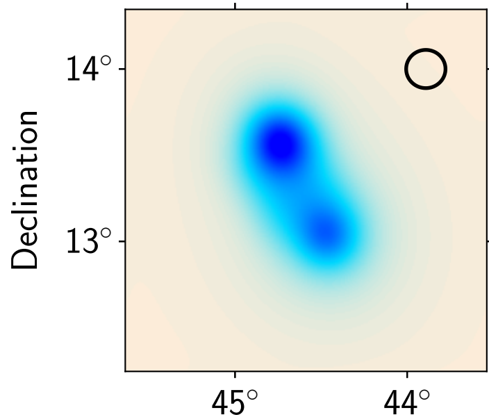
Model: Planck 70 GHz
