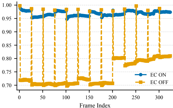
Frame SSIM
