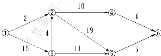
图 6.36 AOE-网
