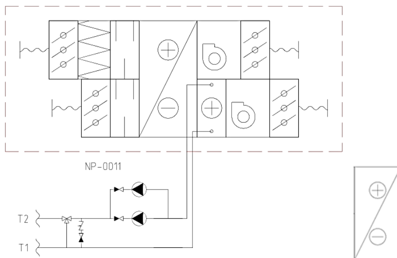
Рис. 3 - Схема установки
