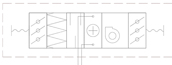
Рис. 1 – Схема установки
