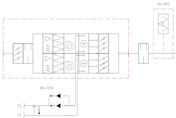
Рис. 2 - Схема установки
