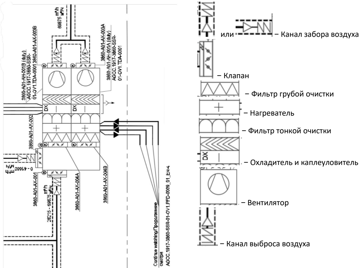
Рис. 5 - Схема установки
