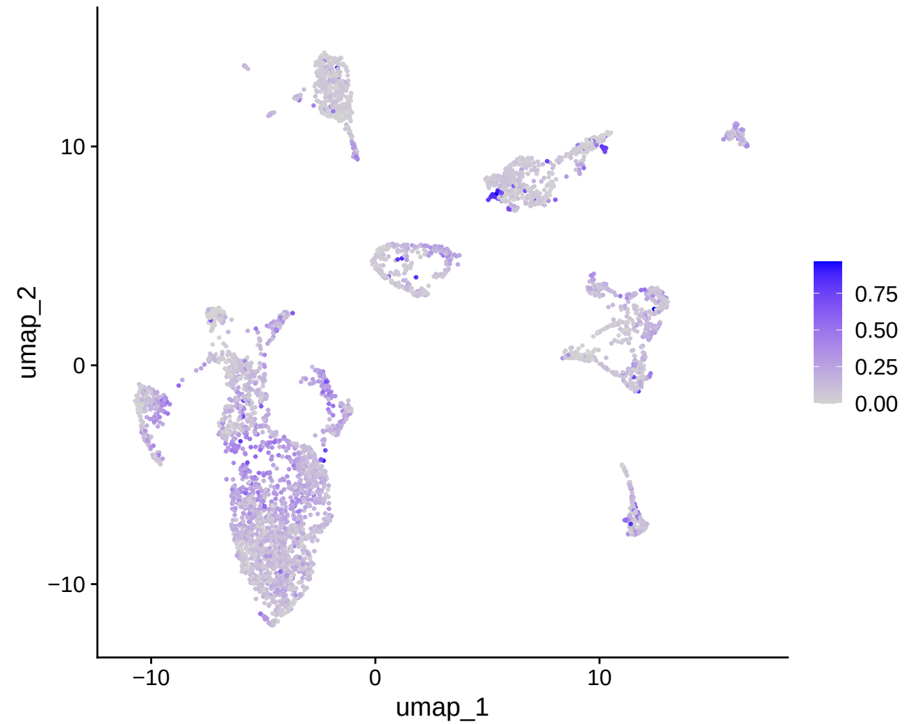
pANN
