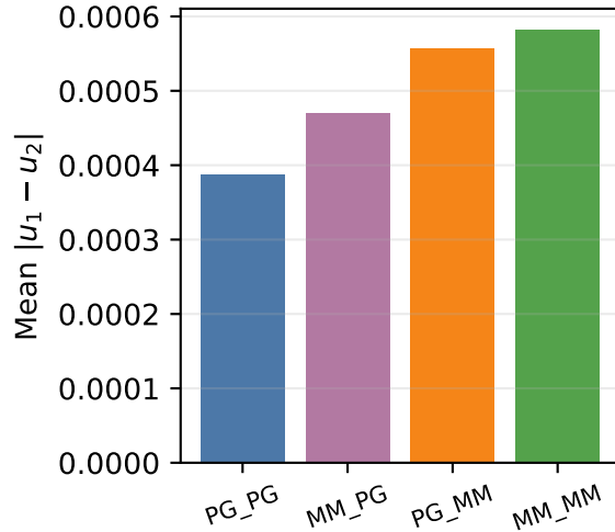
Exploitation gap
