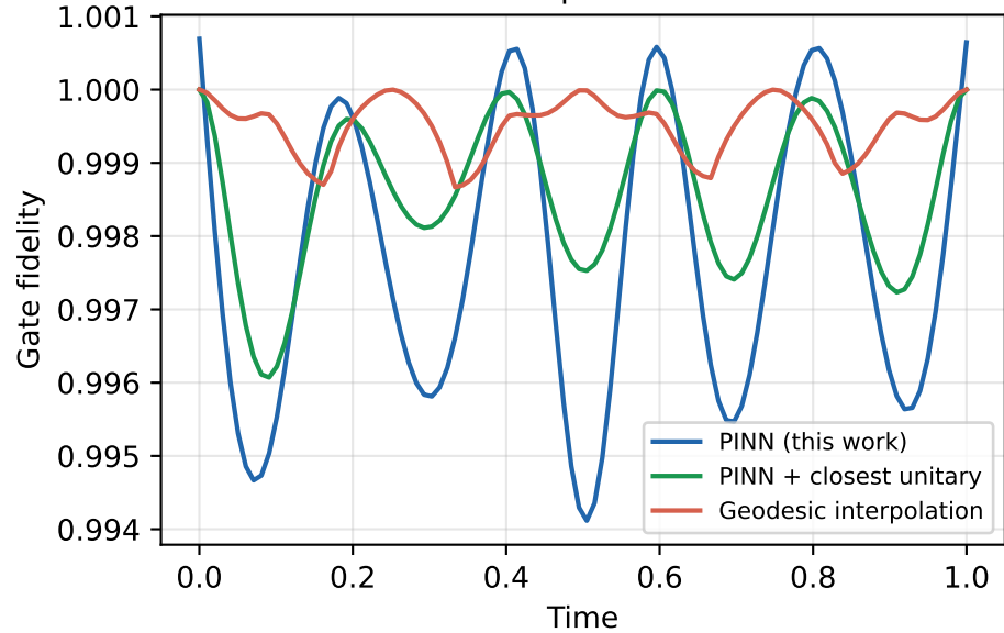
5 qubits
