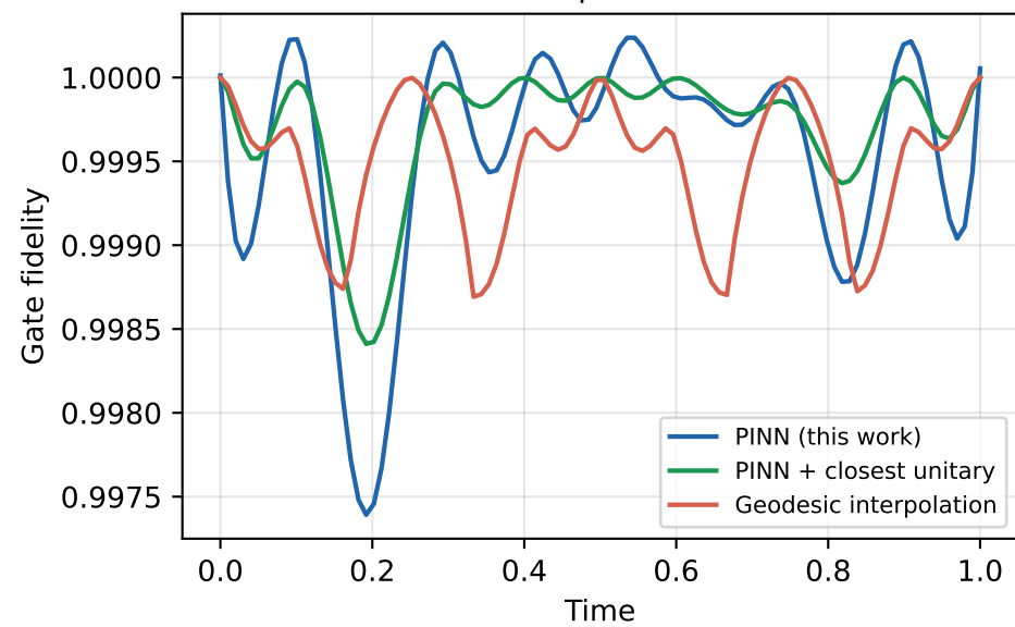
6 qubits
