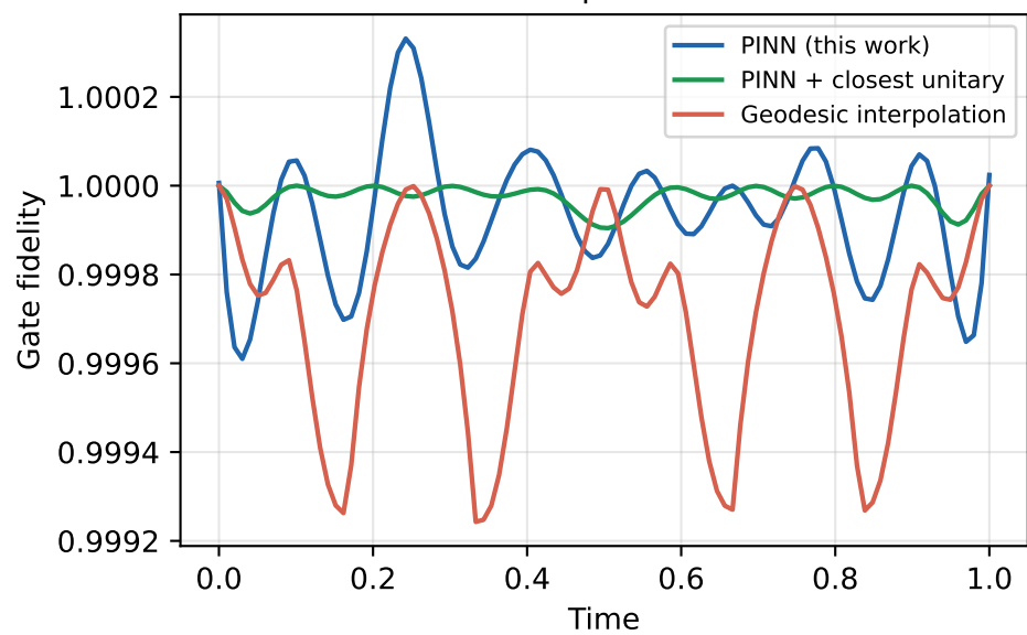
5 qubits
