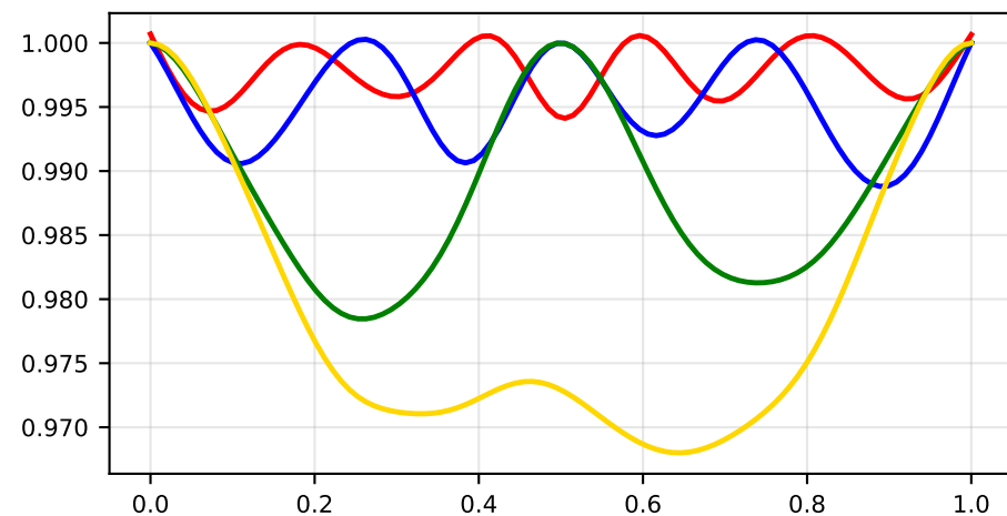
5 Qubits
