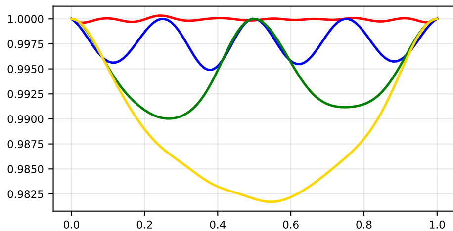
6 Qubits
