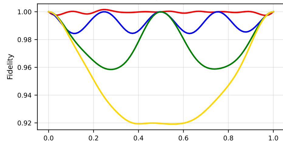
4 Qubits
