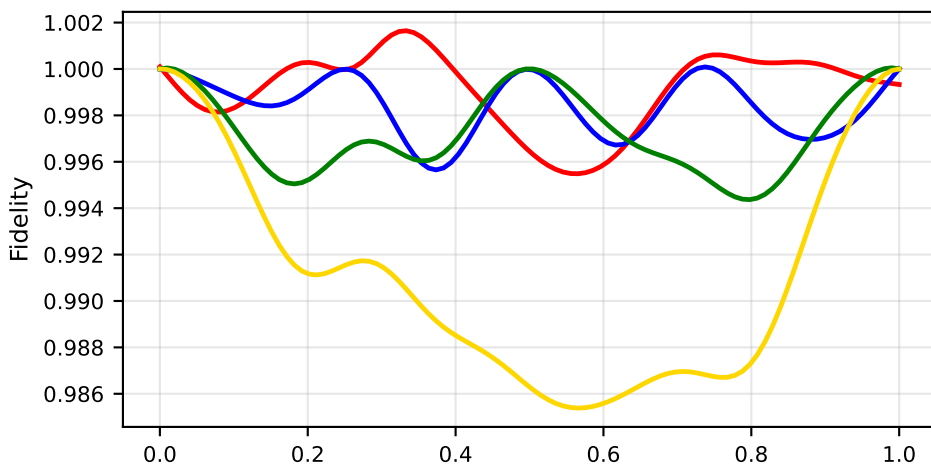
4 Qubits
