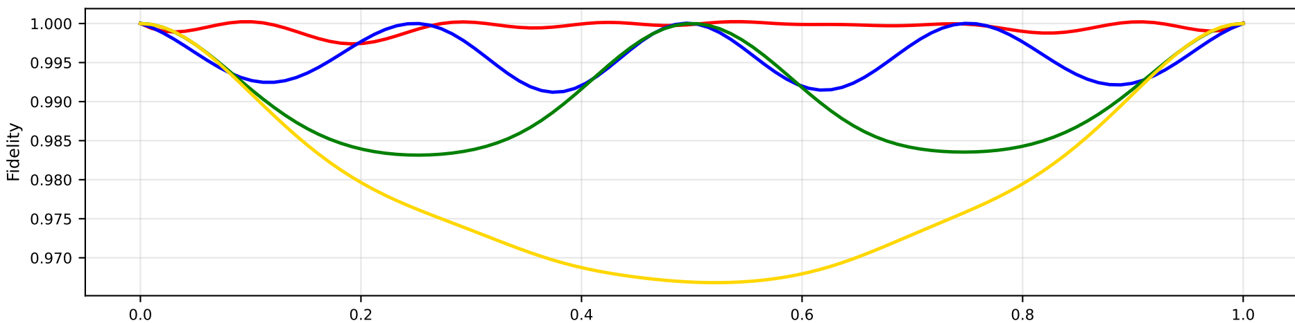
6 Qubits
