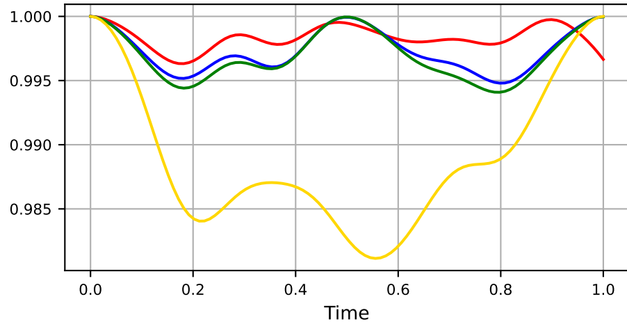
8 Qubits
