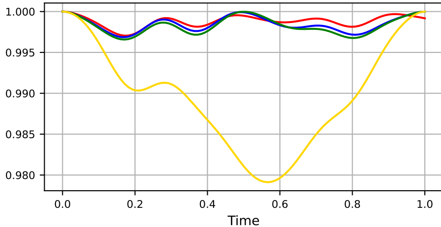
7 Qubits
