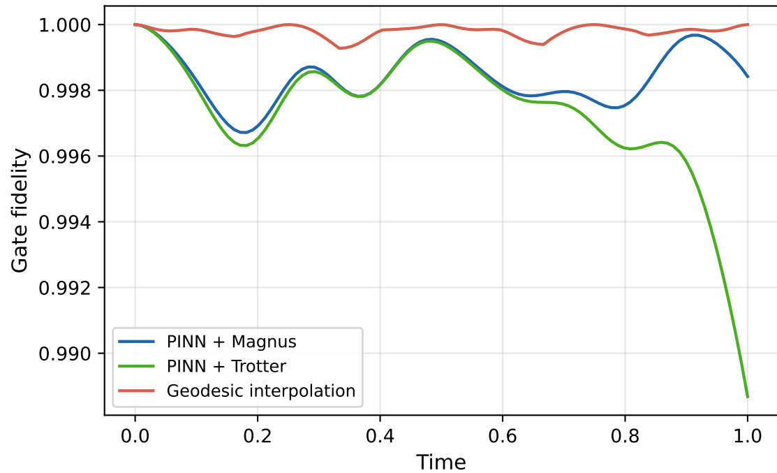
8 qubits
