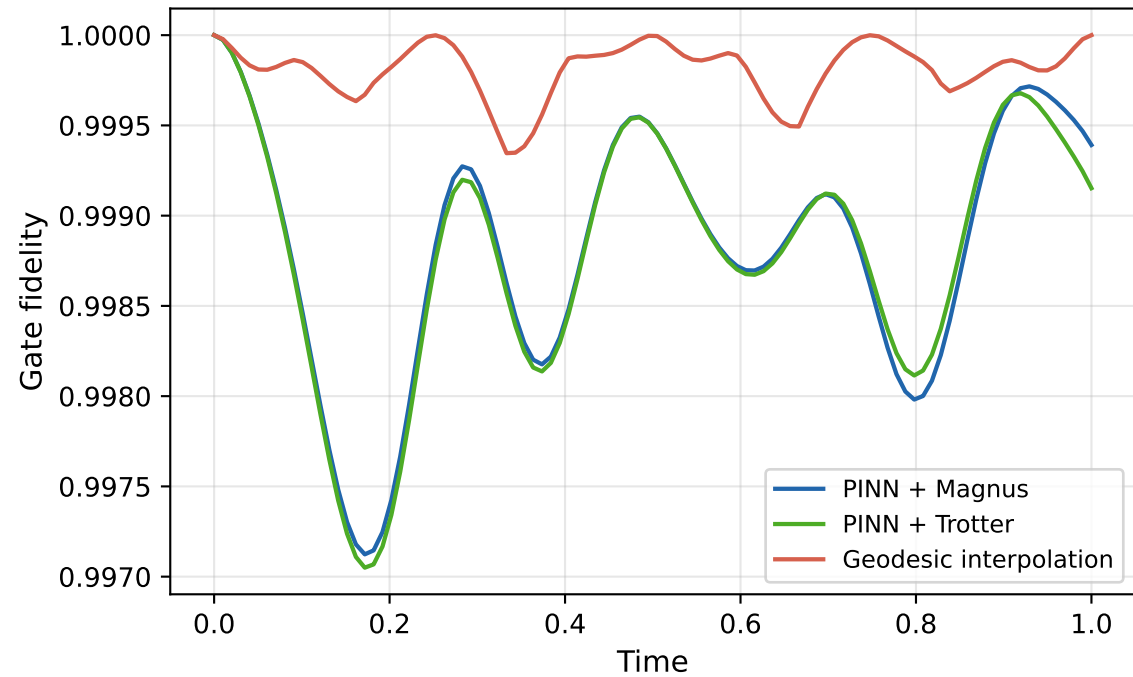
7 qubits
