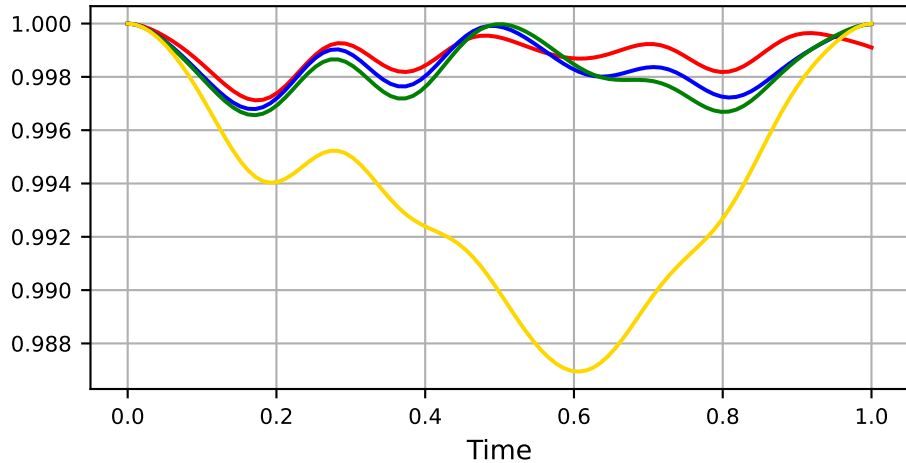
7 Qubits
