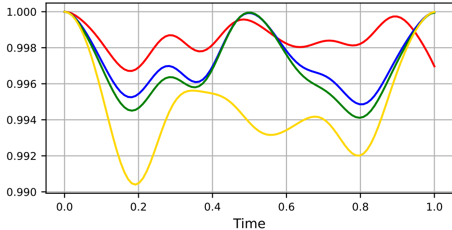
8 Qubits
