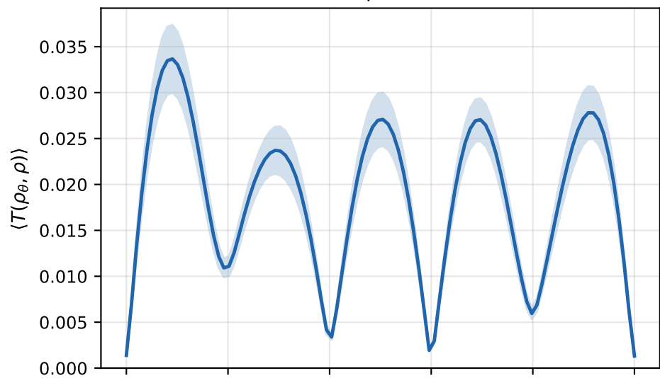
5 qubits
