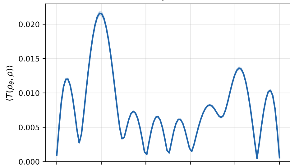
8 qubits
