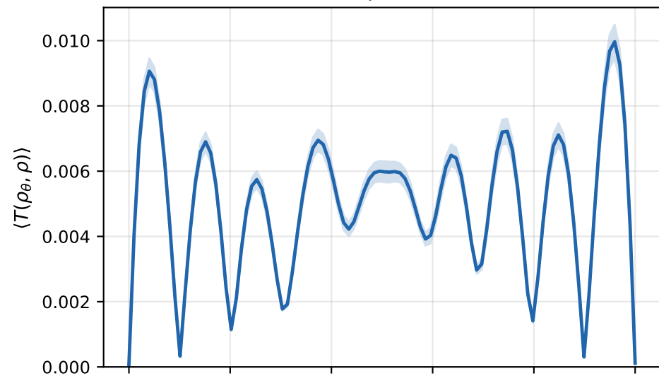
6 qubits
