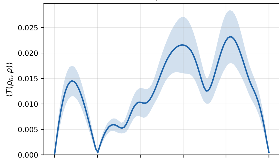
4 qubits
