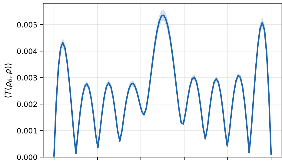
7 qubits
