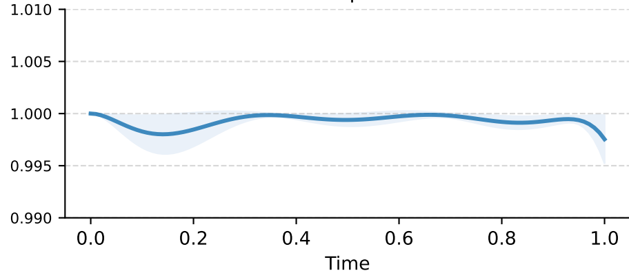
N=8 qubits
