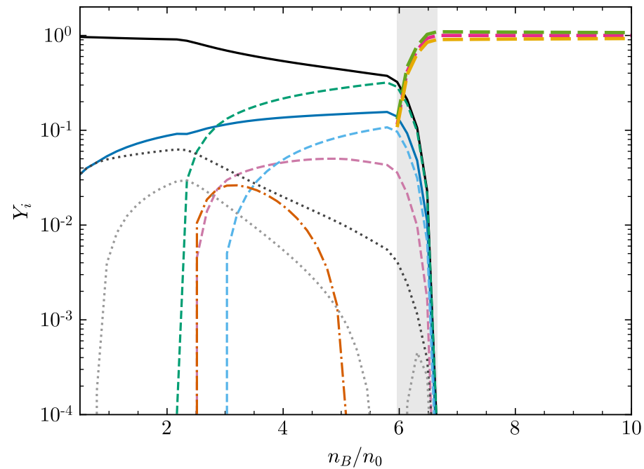
\beta -eq, T=0 MeV, \eta=1
