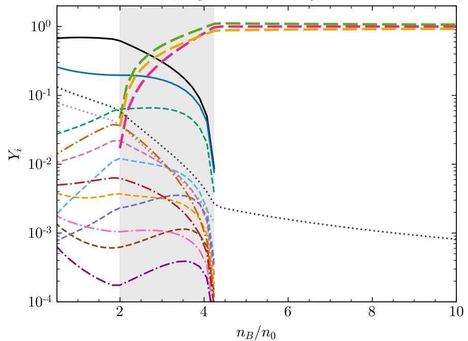
\beta -eq, T=50 MeV, \eta=0.3
