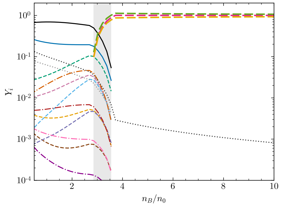
\beta -eq, T=50 MeV, \eta=1
