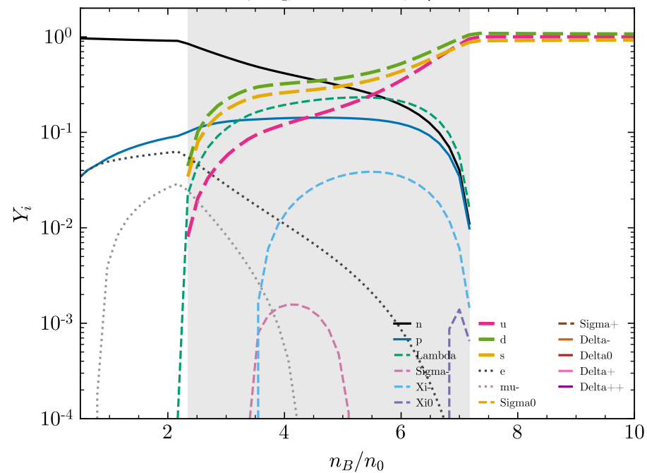
\beta -eq, T=0 MeV, \eta=0.3
