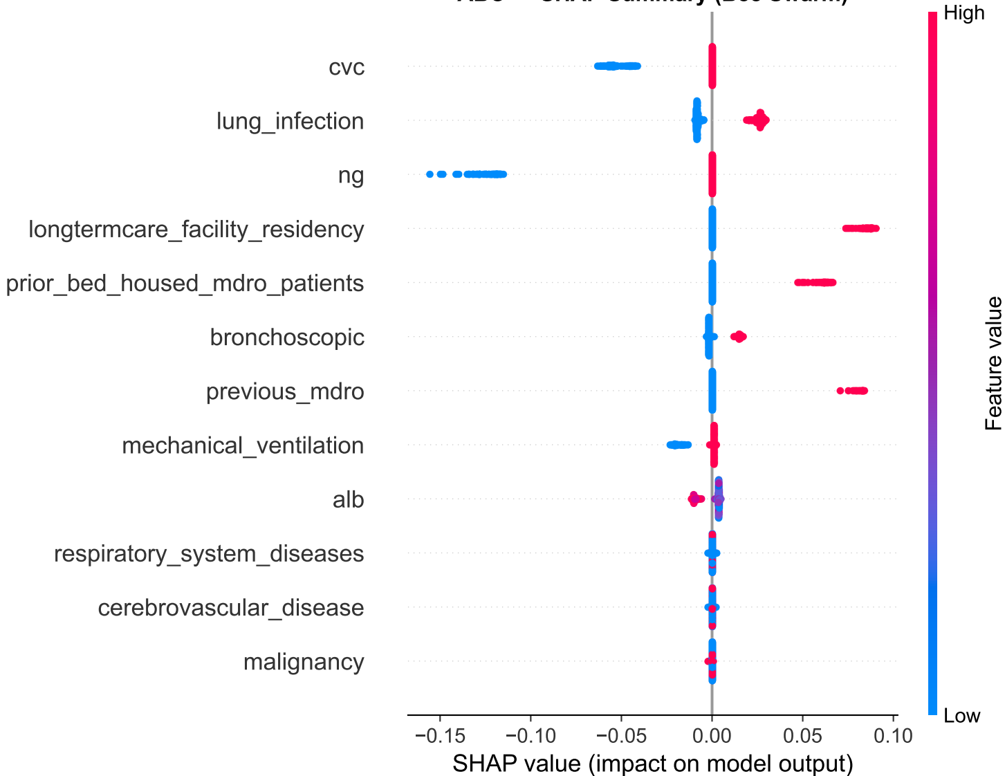
ABC — SHAP Summary (Bee Swarm)
