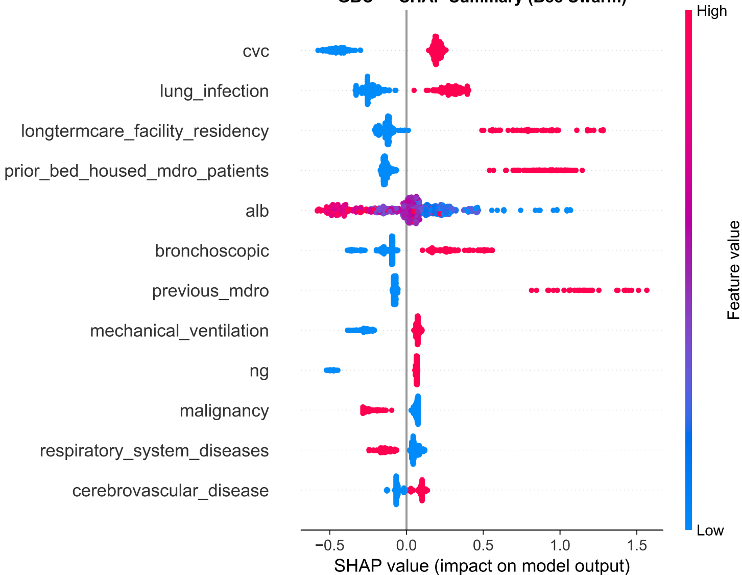
GBC — SHAP Summary (Bee Swarm)
