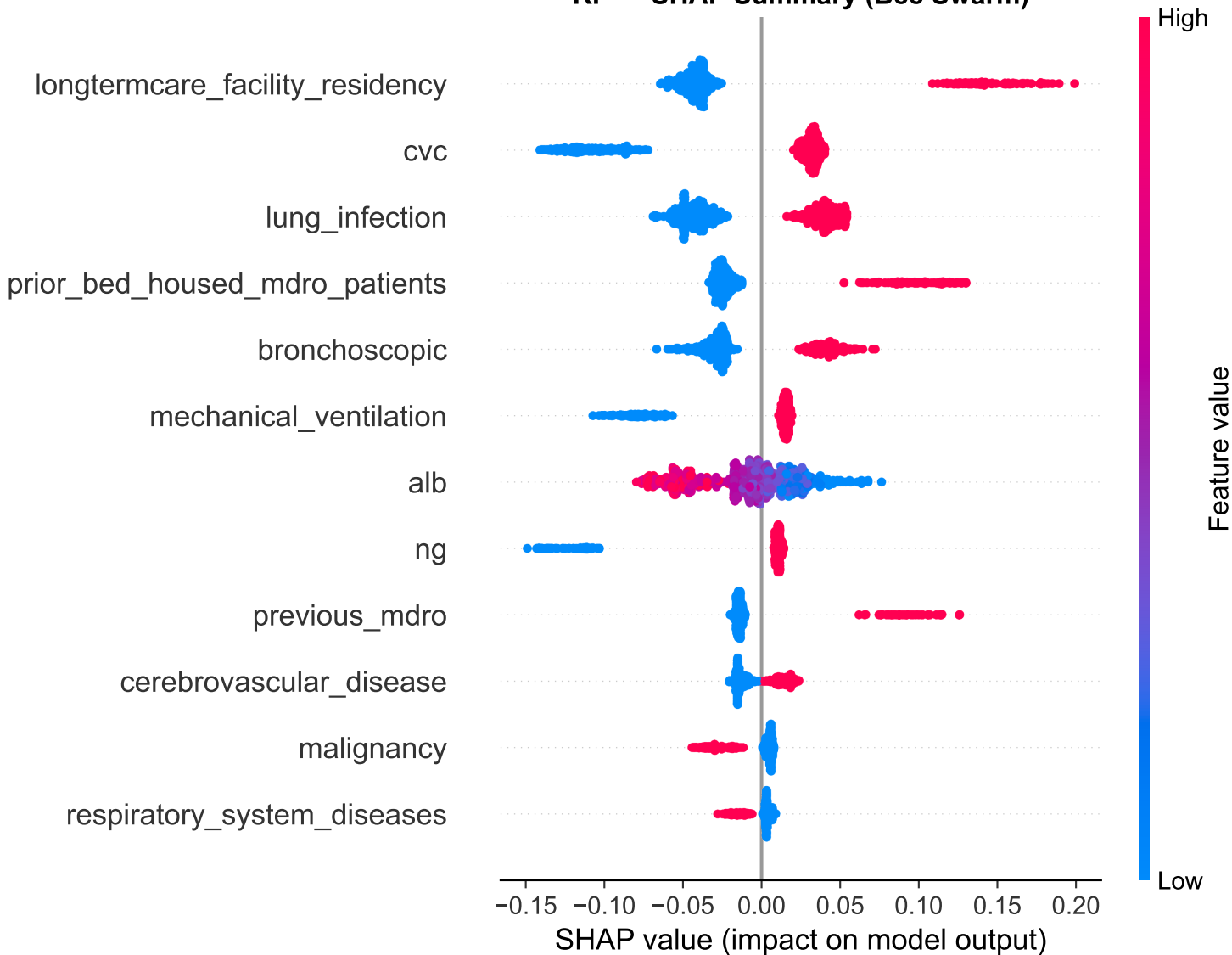
RF — SHAP Summary (Bee Swarm)
