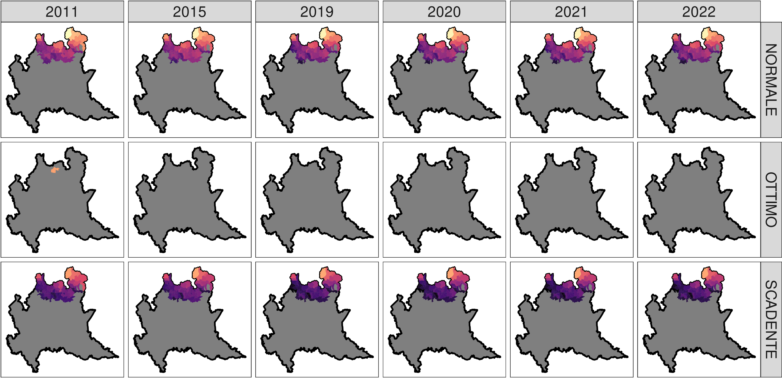
Log prices for Sales of 'Abitazioni_tipiche_dei_luoghi' (normalized)
