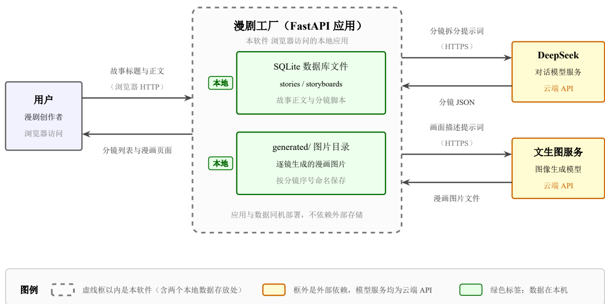
图 2 软件与外部环境关系图
