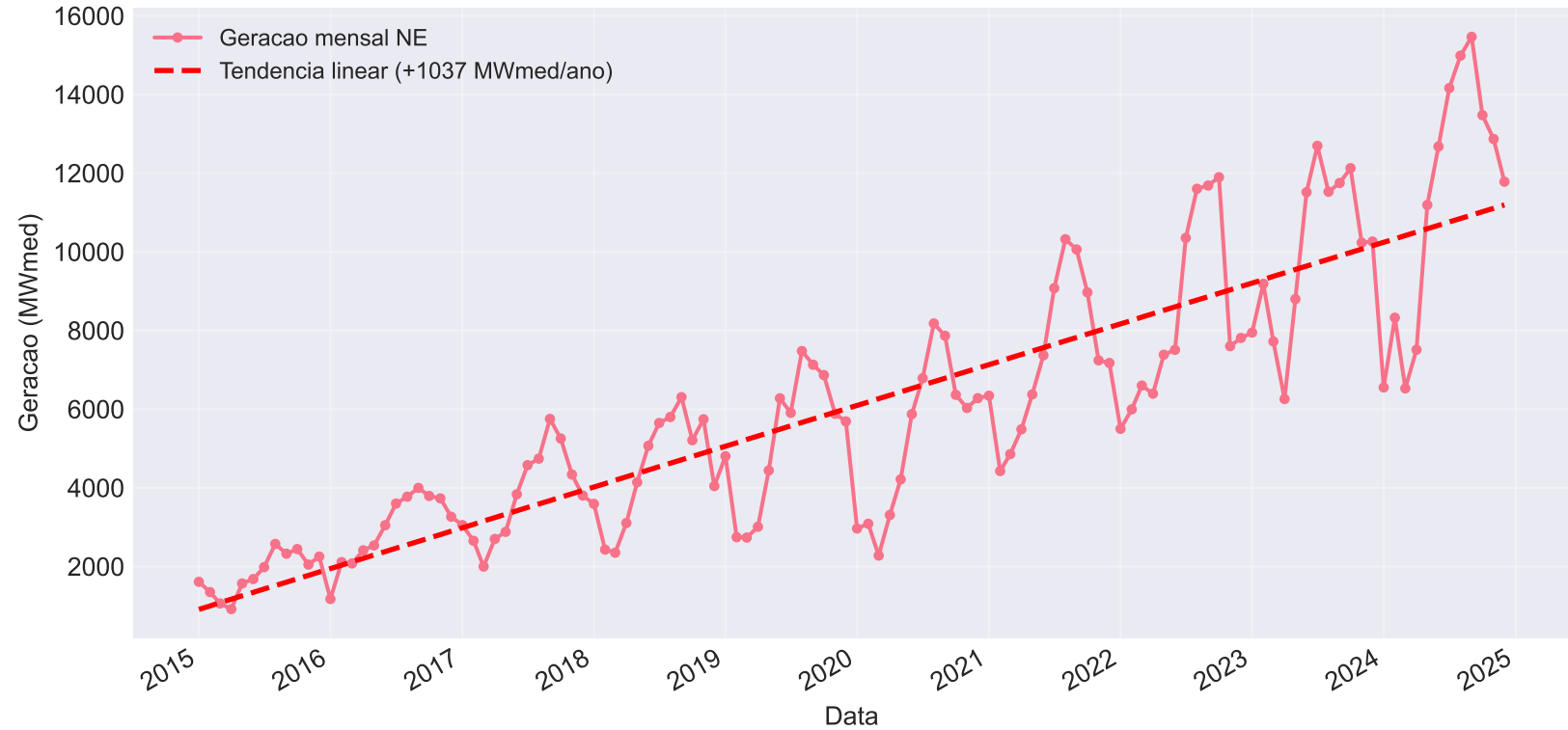
Geracao eolica mensal — Subsistema Nordeste (2015-2024)
