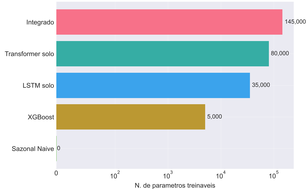
Complexidade dos modelos por parametros
