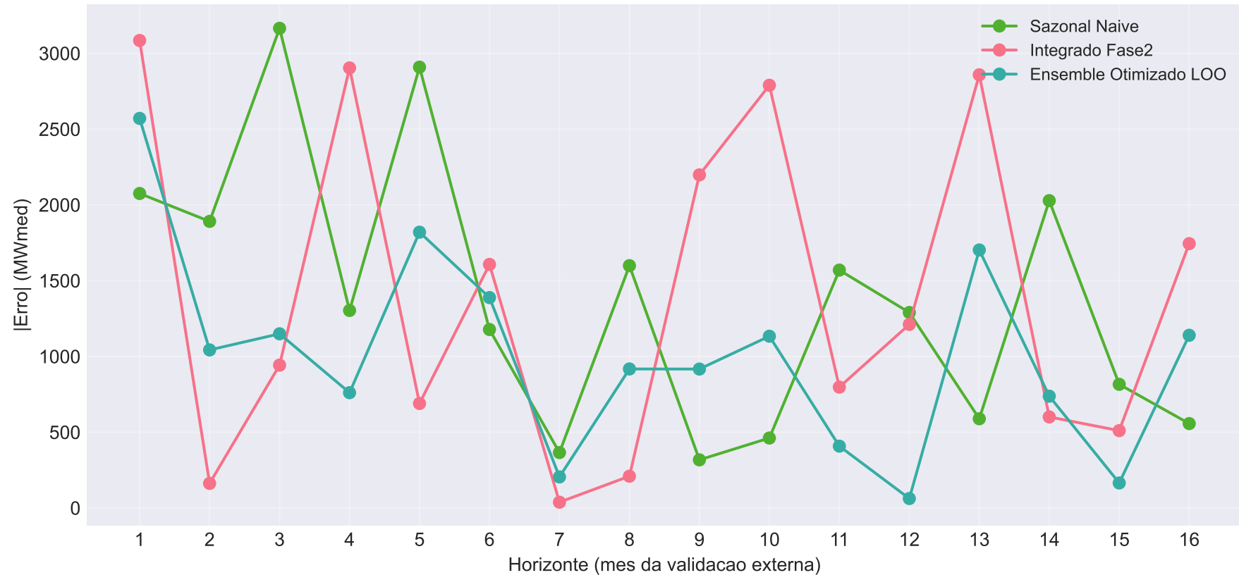
Erro absoluto vs horizonte — inversao de regime Sazonal/Integrado
