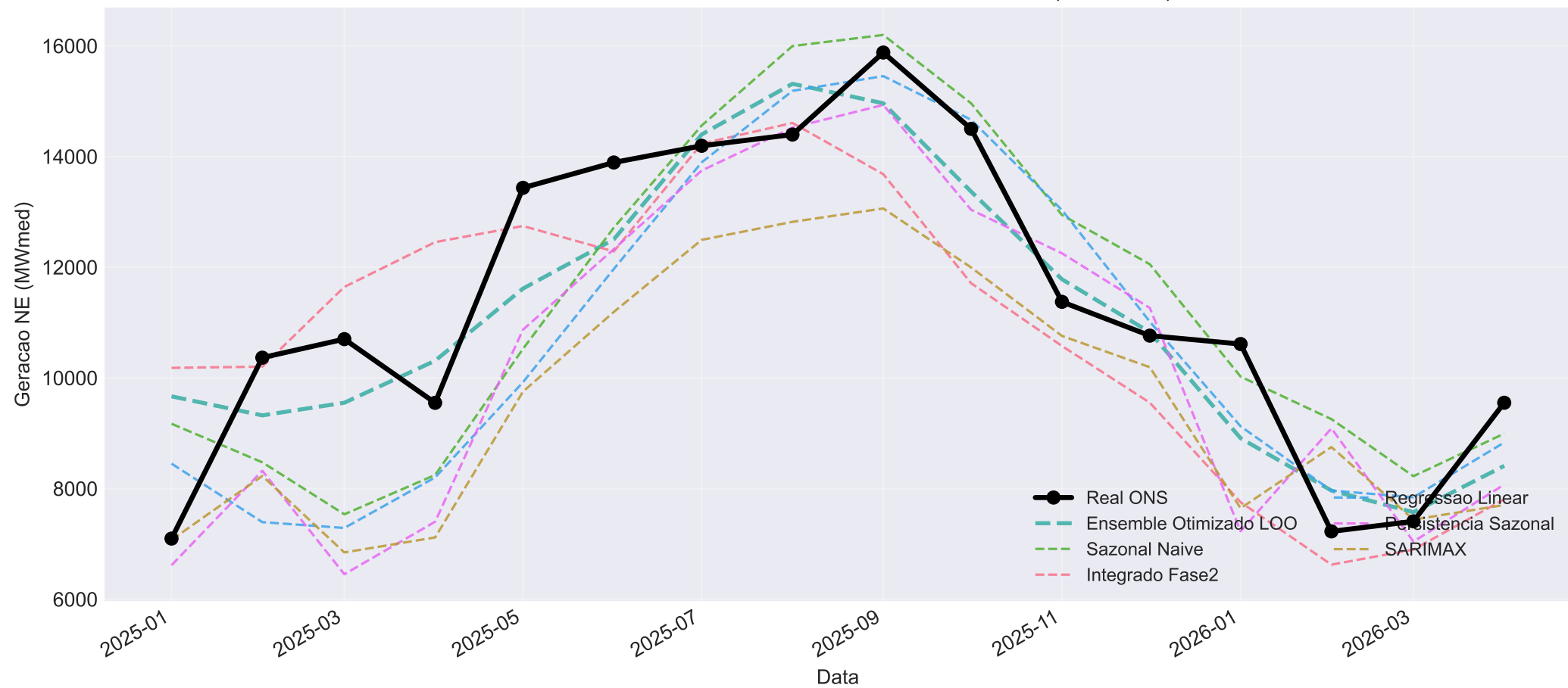
Validacao externa: todos os modelos vs Real ONS (16 meses)
