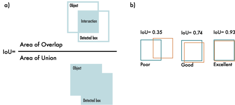
Figure 2.5. Schématisation de l'IoU (figure issue de [20]).
