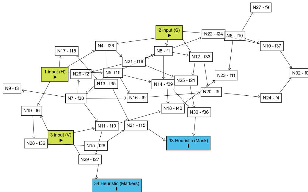
Figure 2.3. Exemple de graphe orienté acyclique de notre propre modèle (voir section 2.3).
