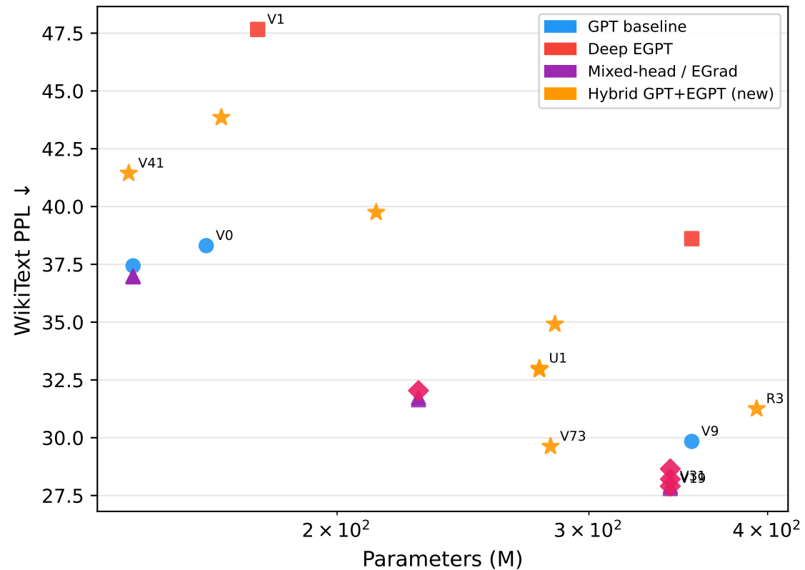
PPL vs. Parameters
