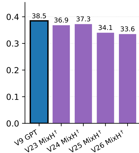
HellaS
