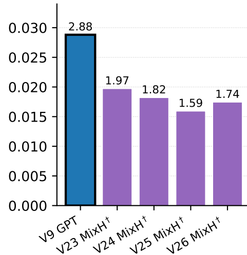
GSM8K
