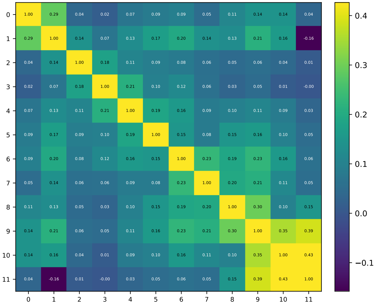
Attn Output Cosine Sim — V0 GPT 12×1 d768
