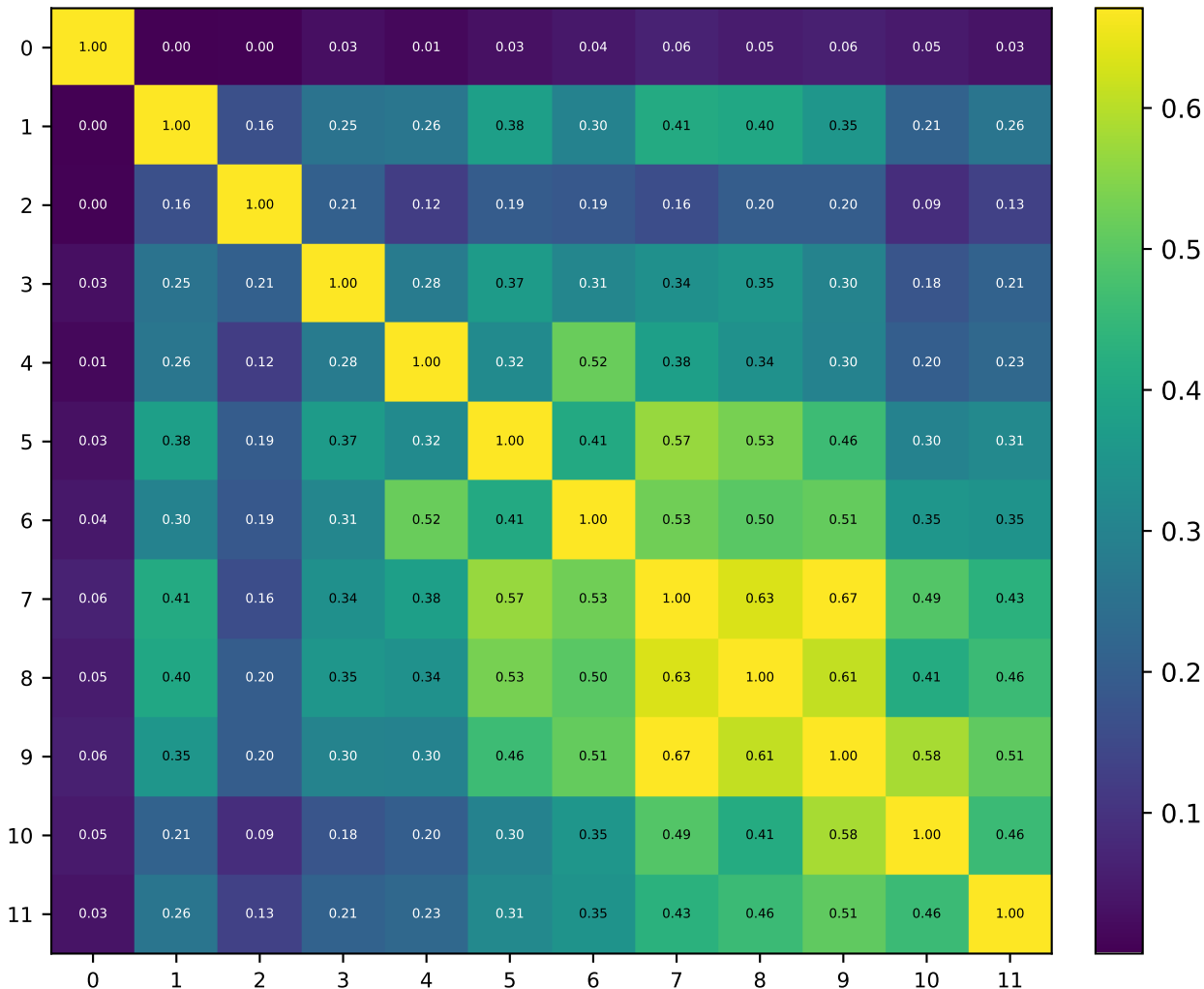
Attn Output Cosine Sim — V1 EGPT 12×1 d768
