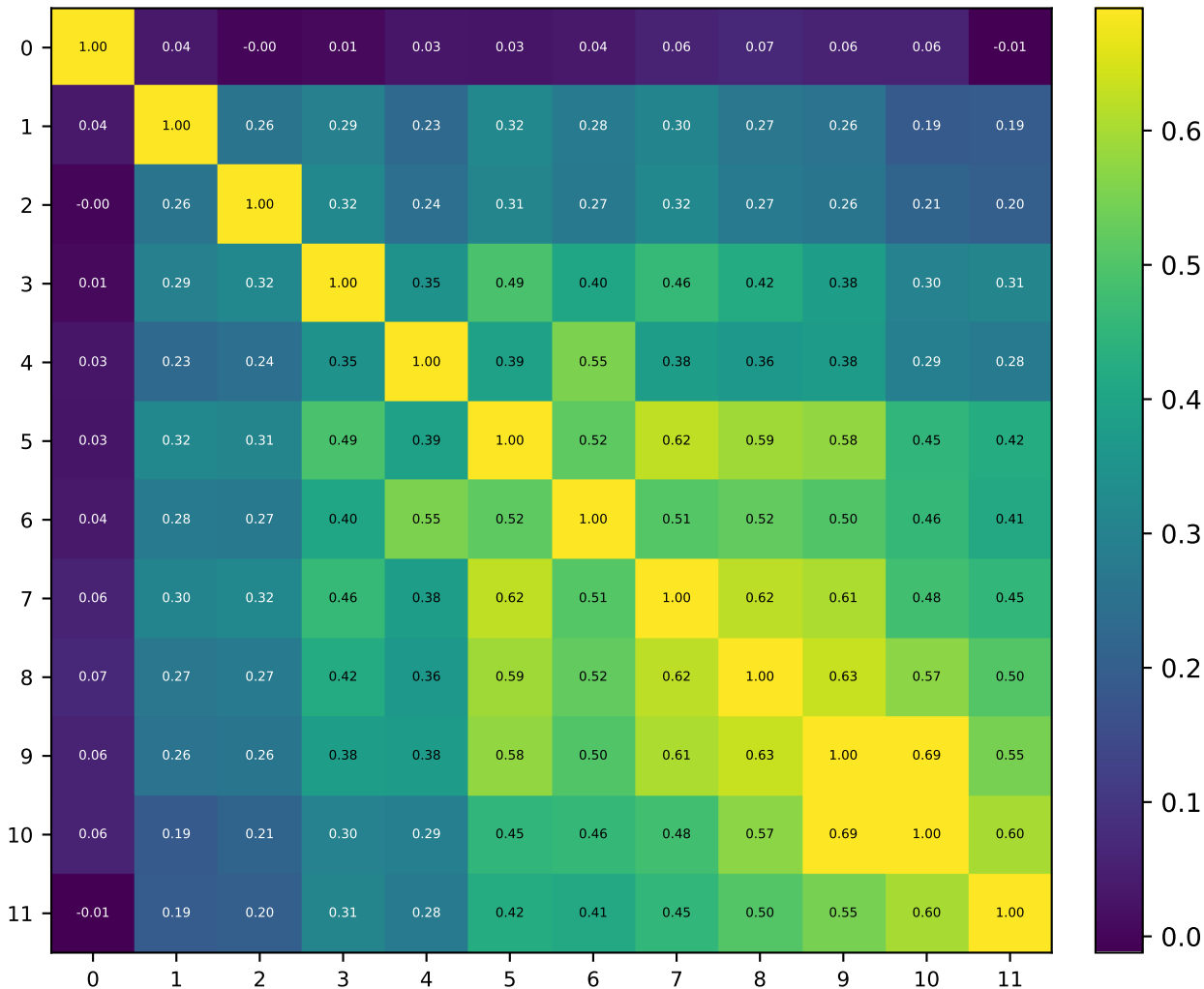
Attn Output Cosine Sim — V39 EGPT +cosreg
