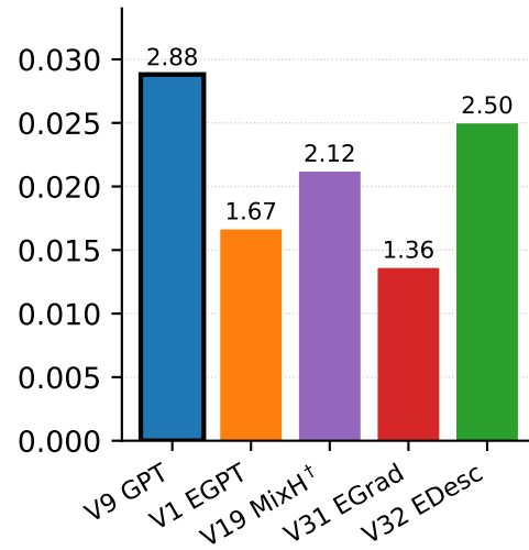
GSM8K
