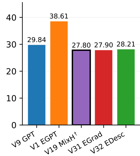
PPL ↓
