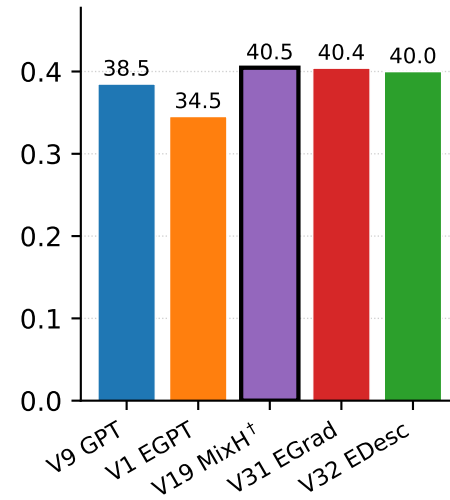
HellaS
