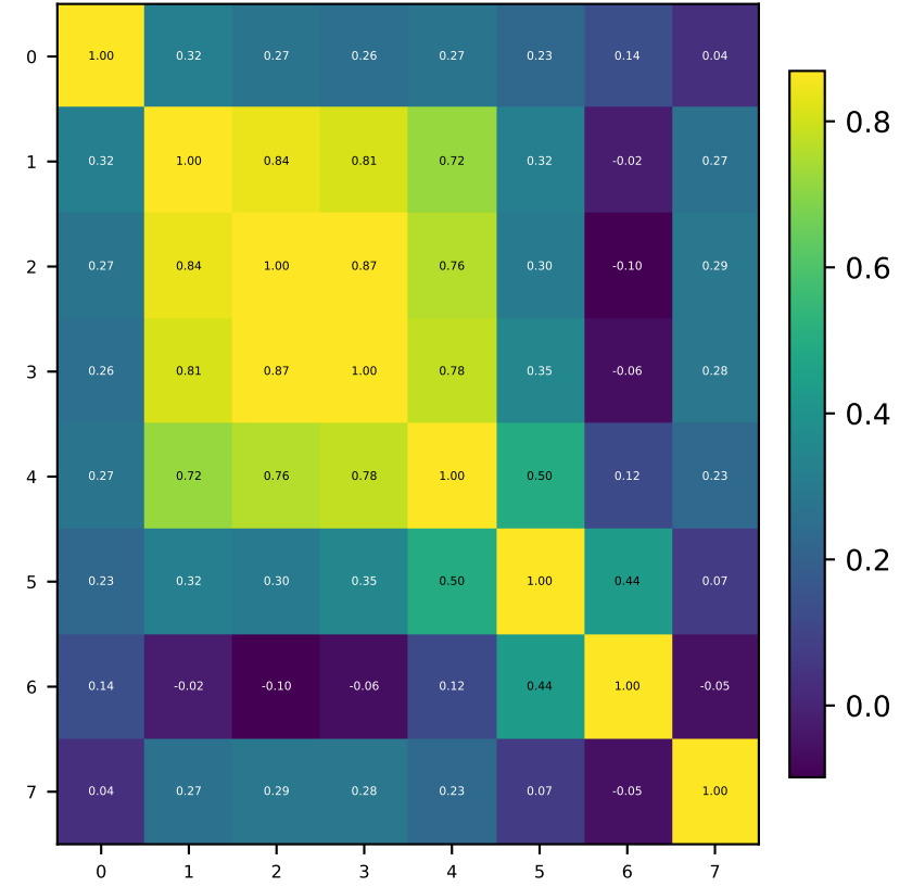
proj_mlp(FFN)
