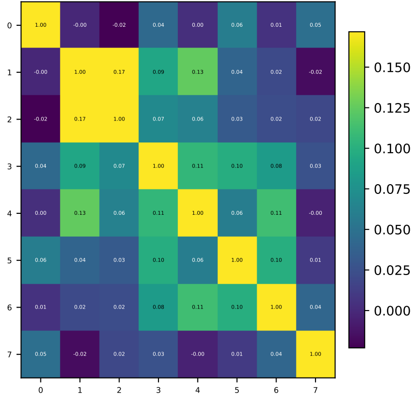
proj_attn(attn)
