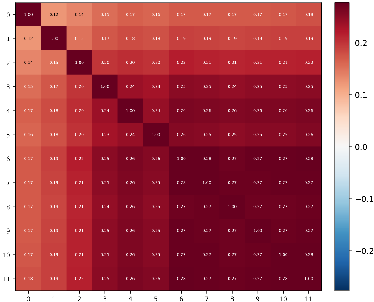
Weight Cosine Similarity — V0 GPT 12×1 d768
