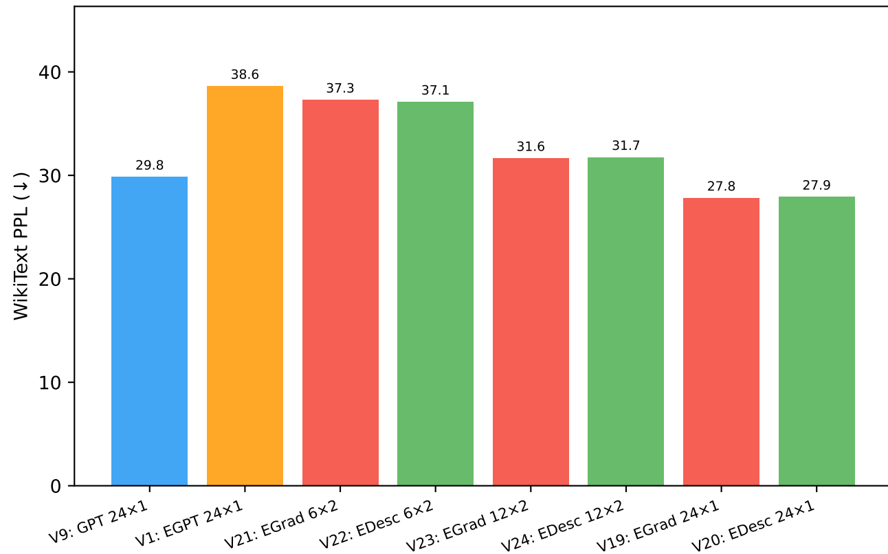
WikiText PPL (↓)
