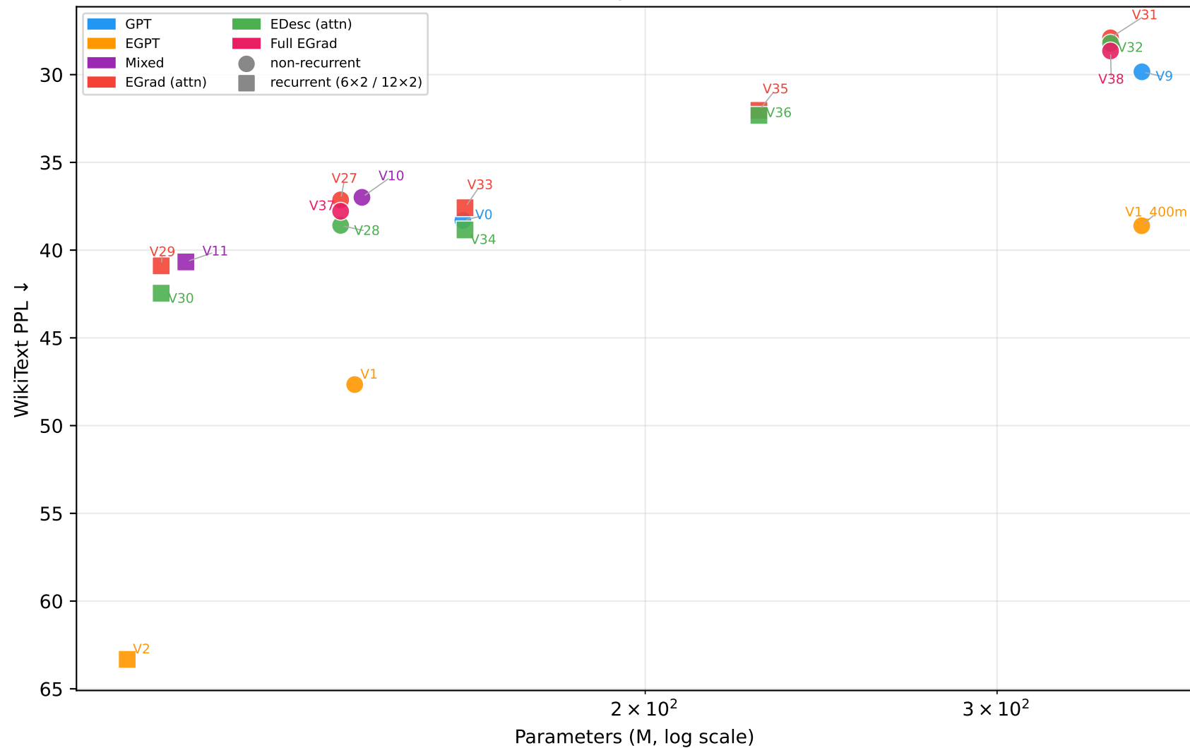
WikiText PPL ↓ vs Parameters (M, log scale) — True EGrad/EDesc (V27-V36)
