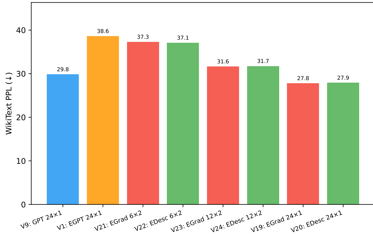
WikiText PPL (↓)
