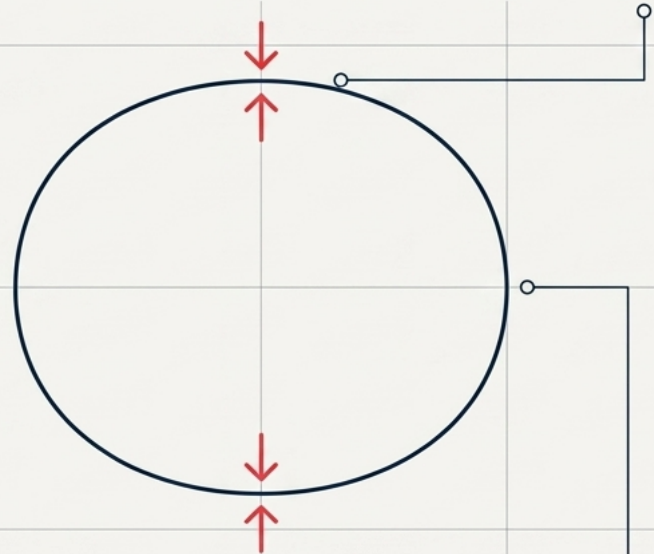
Earth's Actual Shape
