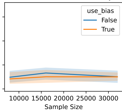
Env=SC-PermExDc-v0; Delay=6
