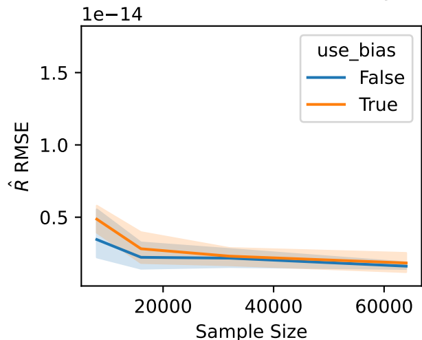
Env=CC-PermExDc-v0; Delay=2
