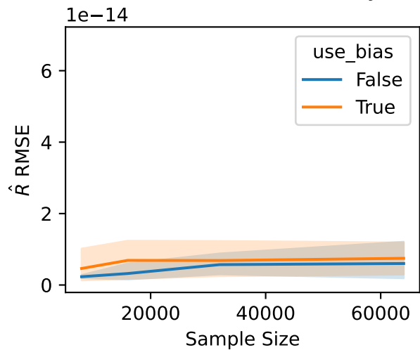
Env=SC-ShuntDc-v0; Delay=2
