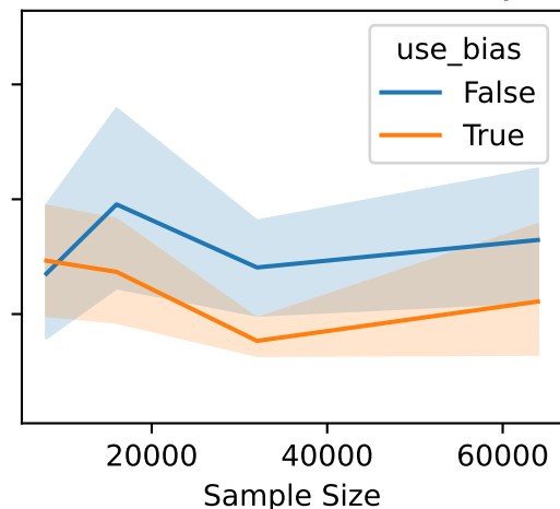
Env=CC-PermExDc-v0; Delay=6
