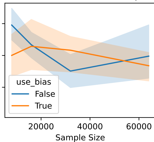
Env=CC-ShuntDc-v0; Delay=6
