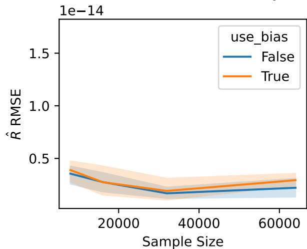
Env=CC-ShuntDc-v0; Delay=2
