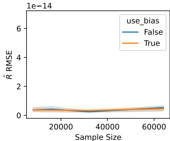
Env=SC-PermExDc-v0; Delay=2
