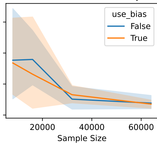
Env=SC-ShuntDc-v0; Delay=6
