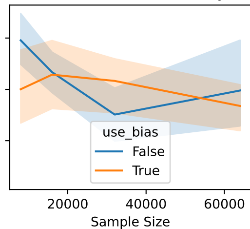
Env=CC-ShuntDc-v0; Delay=6
