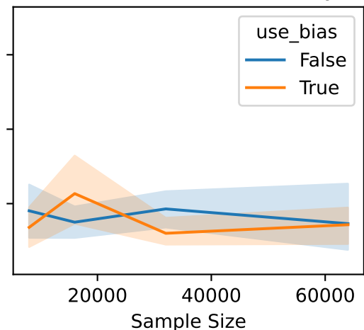
Env=CC-PermExDc-v0; Delay=4
