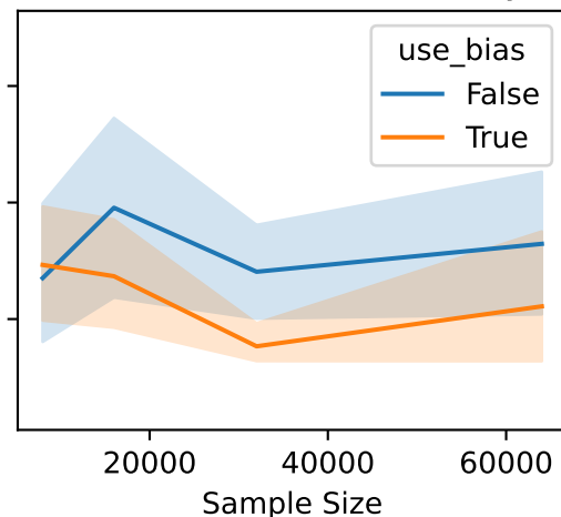
Env=CC-PermExDc-v0; Delay=6
