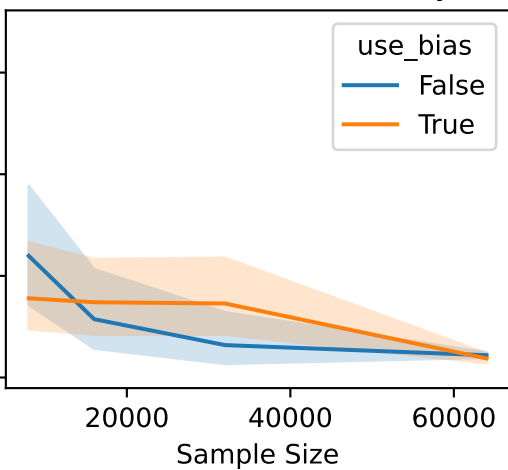
Env=SC-ShuntDc-v0; Delay=4
