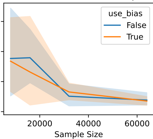
Env=SC-ShuntDc-v0; Delay=6
