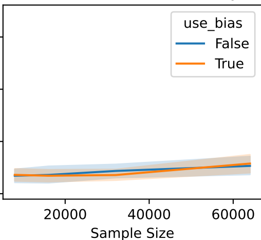
Env=SC-PermExDc-v0; Delay=4
