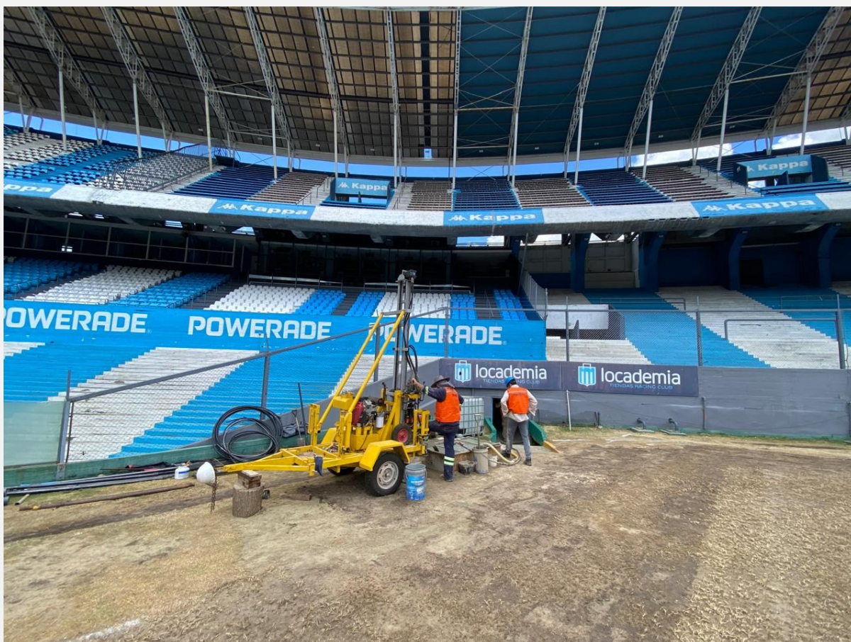
Inicio de los trabajos de perforación para la explotación de agua en la última semana de diciembre 2024
