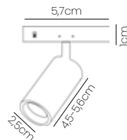
mini spot led para trilho PIÙ BELLA Ref: SKY-353
