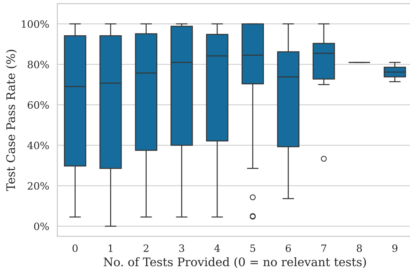
date-fns
