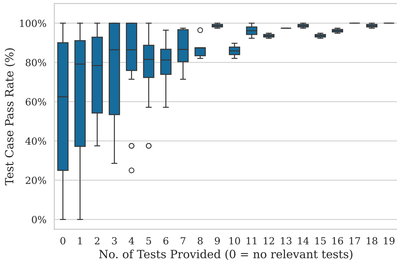
directus
