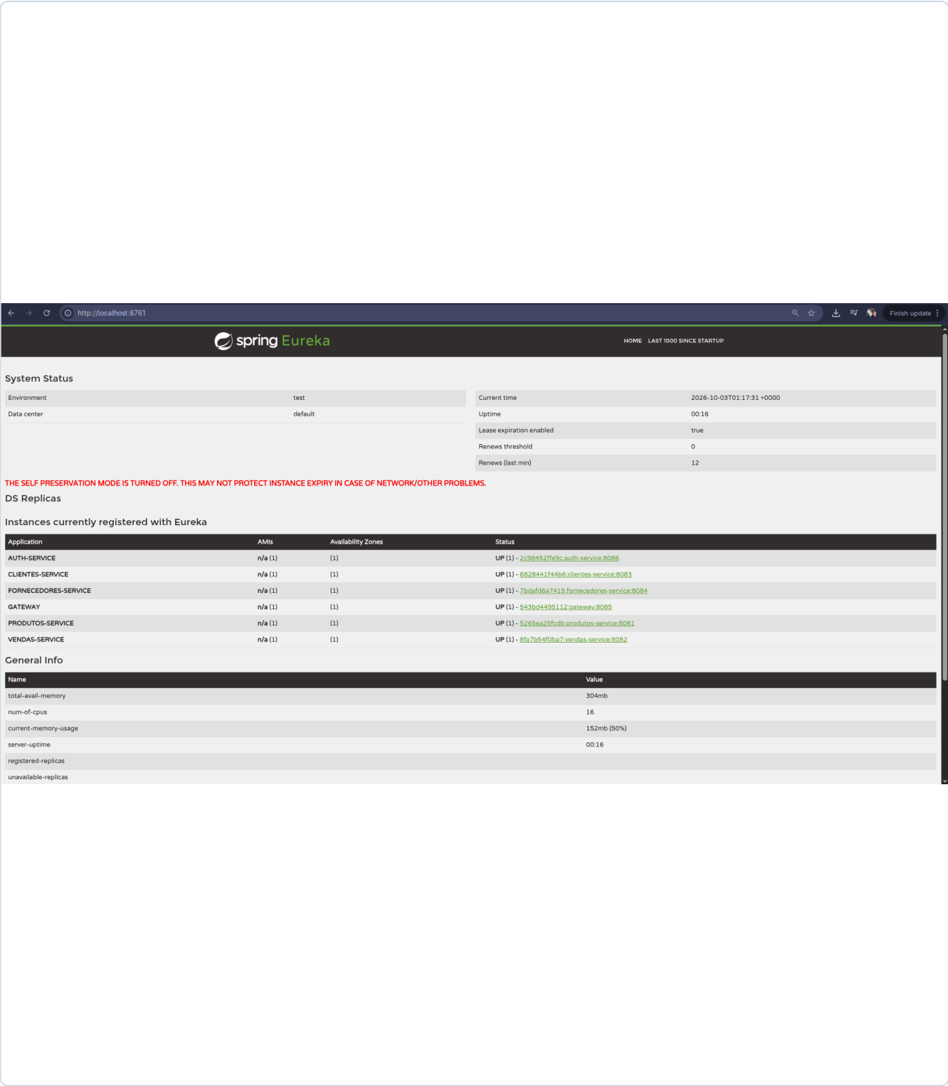
Figura 1 — Registro do produtos-service no Eureka.
