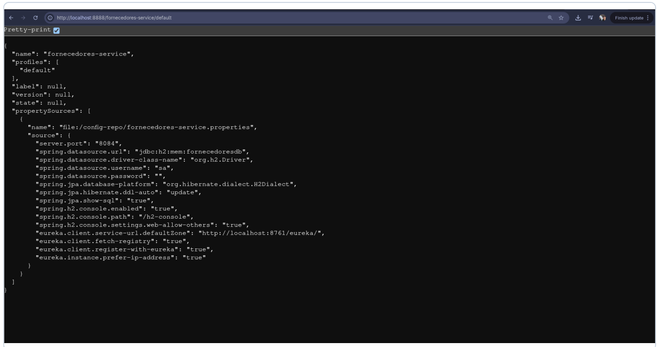
Figura 7A — Propriedades do serviço fornecidas pelo Config Server.
