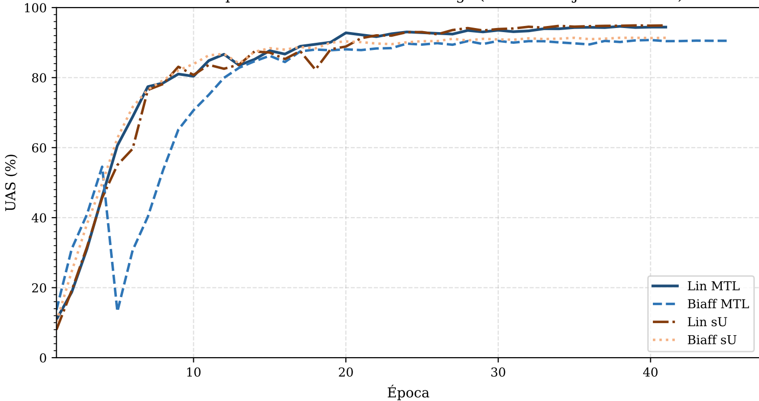
Curvas de Aprendizizado — BERTimbau Large (UAS no conjunto de teste)
