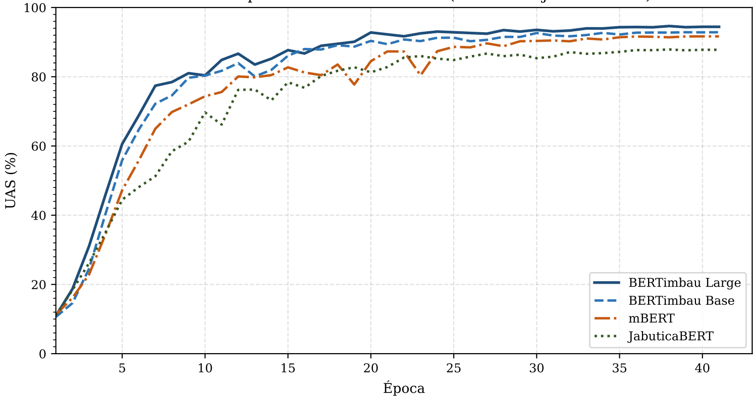
Curvas de Aprendizado — Linear MTL (UAS no conjunto de teste)
