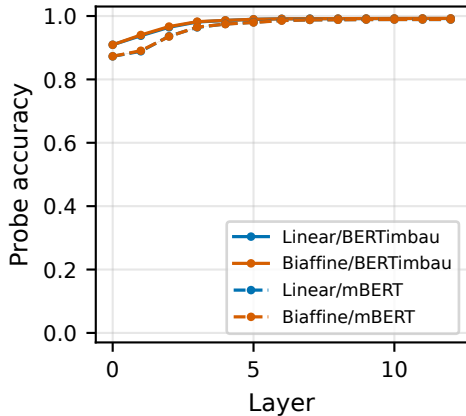
UPOS
